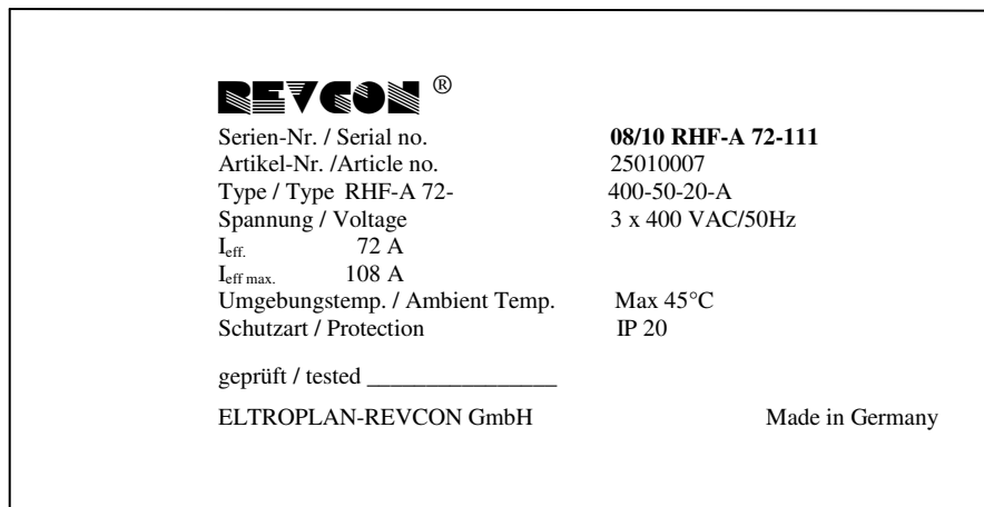
Abbildung 1: REVCON® RHF Typenschild
