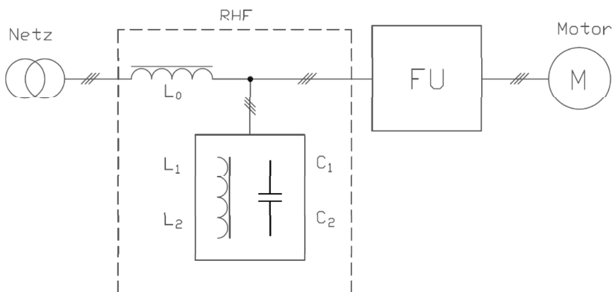
Abbildung 3: Funktionsprinzip RHF
