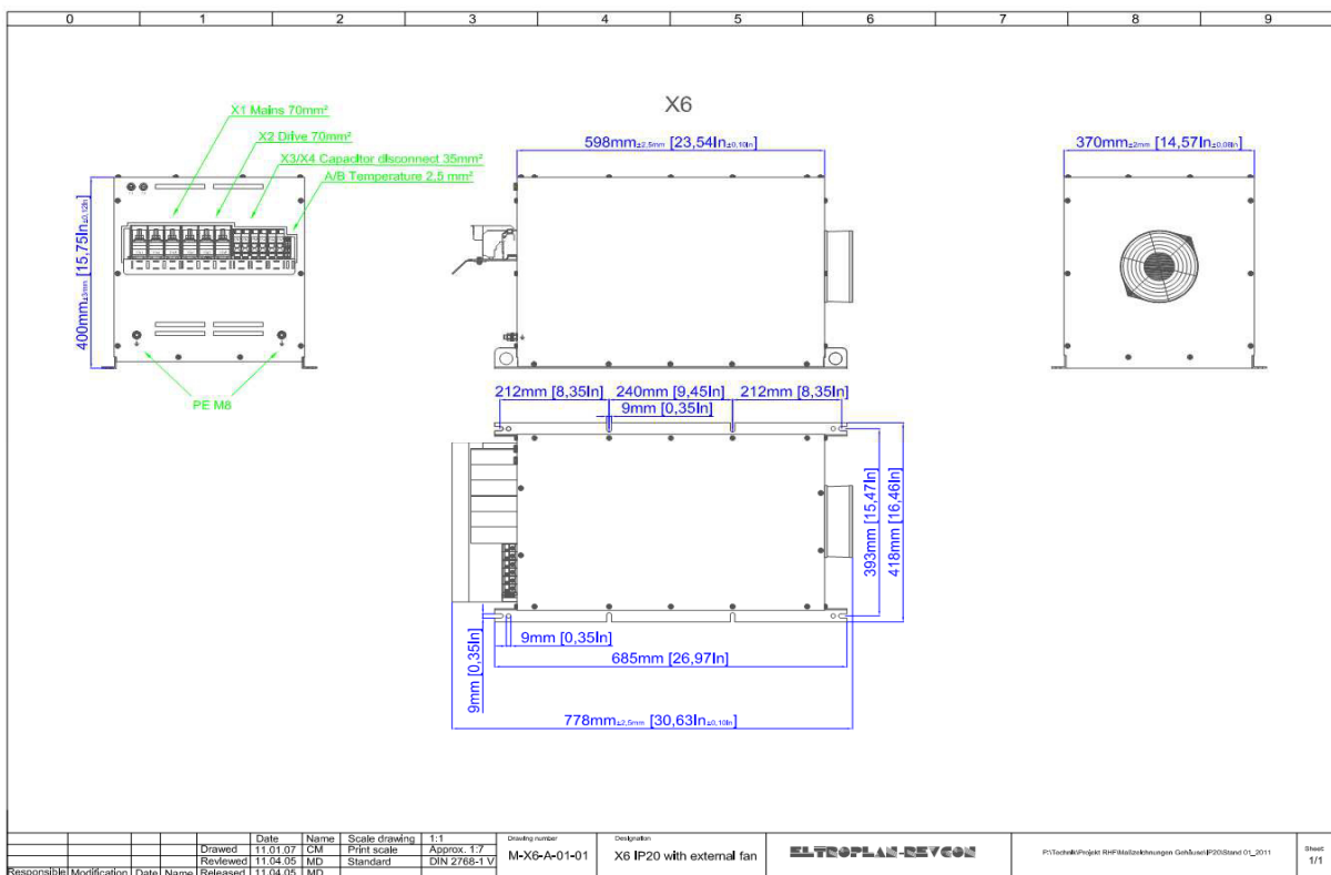
Abbildung 19: Maßbild Bauform X6 Lüfter außen
