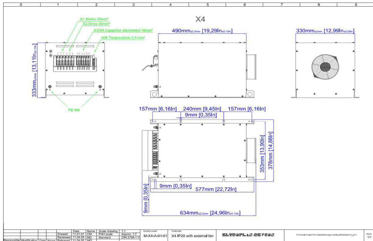
Abbildung 15: Maßbild Bauform X4 Lüfter außen
