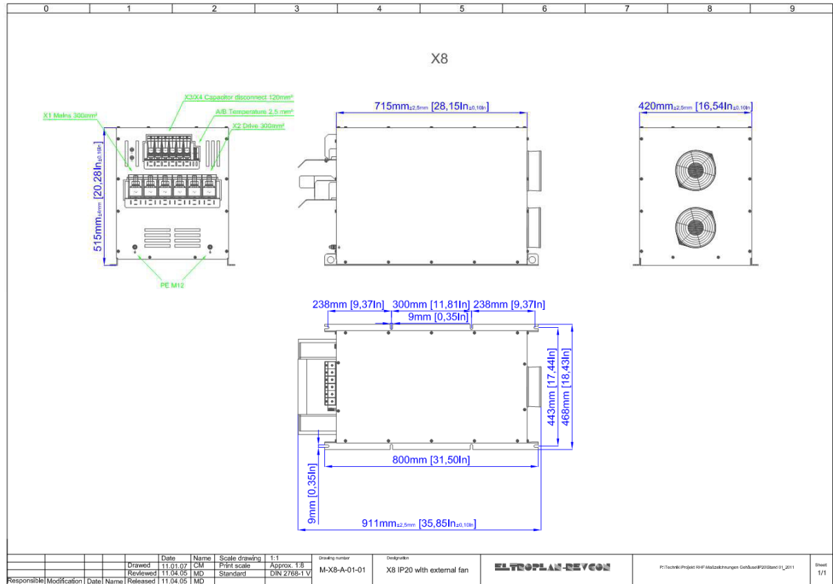
Abbildung 23: Maßbild Bauform X8 Lüfter außen
