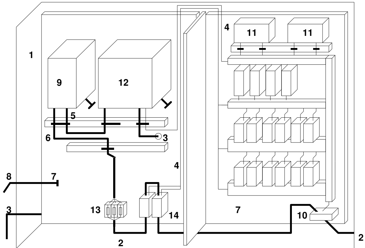
Abbildung 31: EMV-gerechter Schaltschrank
