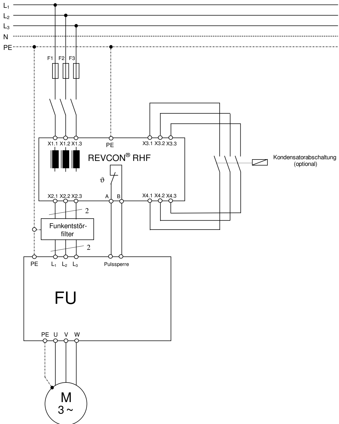
Abbildung 27: Anschluss des Filtermoduls REVCON® RHF an einen Antriebsregler
