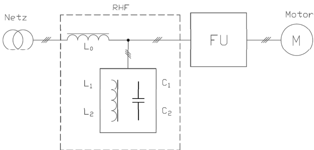
Abbildung 26: Funktionsprinzip RHF
