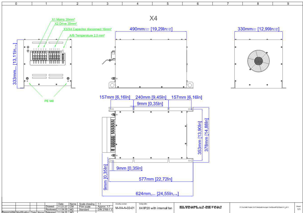
Abbildung 14: Maßbild Bauform X4 Lüfter innen
